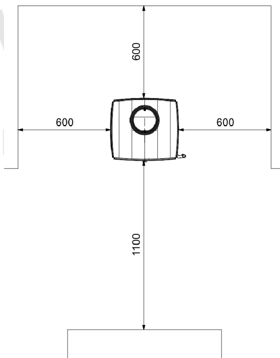
FIG. 7 DISTANZE DI SICUREZZA SENZA LO SCUDO PROTETTORE (mm)
