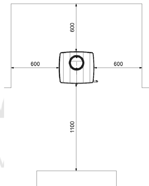
FIG. 7 DISTANCE DE SÉCURITÉ SANS PLAQUE DE PROTECTION ARRIÈRE (mm)
