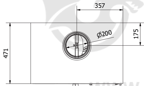
G-G ( 1 : 10 )
