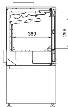
C-C ( 1 : 10 )
