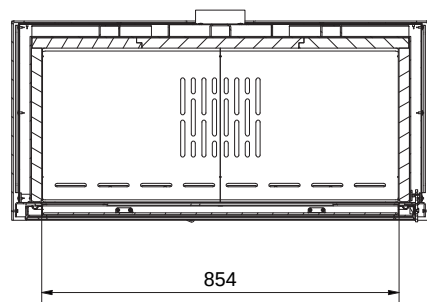
D-D ( 1 : 10 )
