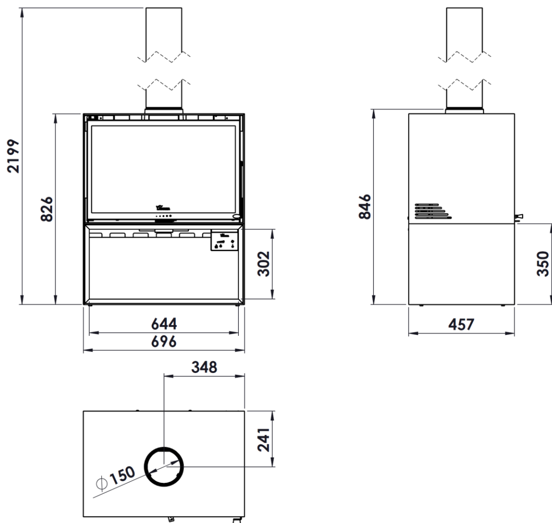
Figura nº1 - Dimensiones en mm del aparato BAIONA 700
