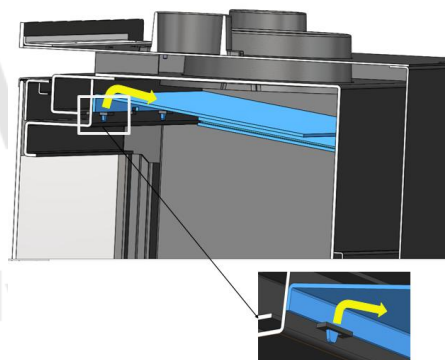
Figura n°24 - Desmontaje del deflector de chapa superior.
