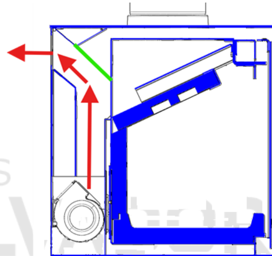
Figura n°16 - Recorrido del aire caliente con canalización
