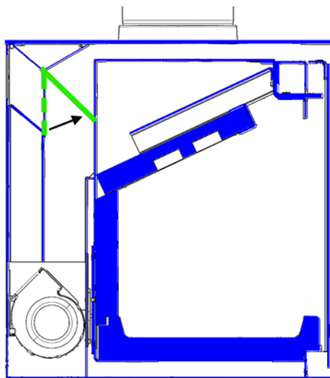
Figura n°15 - Empujar la chapa interior hasta hacer tope
