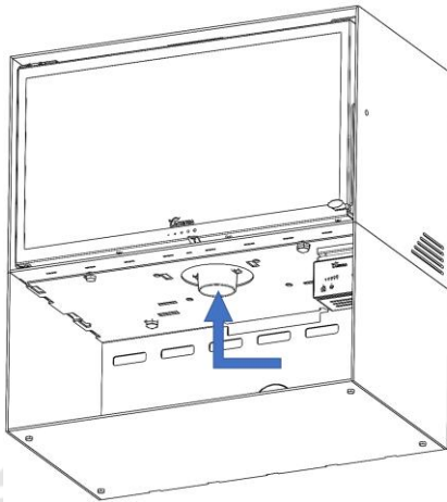
Figura n°5 - Conducción de aire para cámara de combustión
