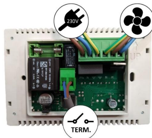
Figura n°7 - Conexiones a realizar en el potenciómetro
