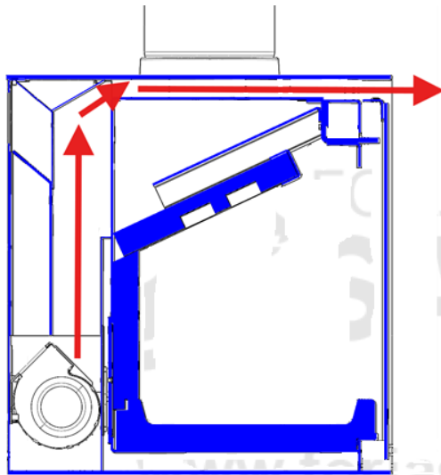
Figura n°14 - Recorrido del aire caliente sin canalizaciones
