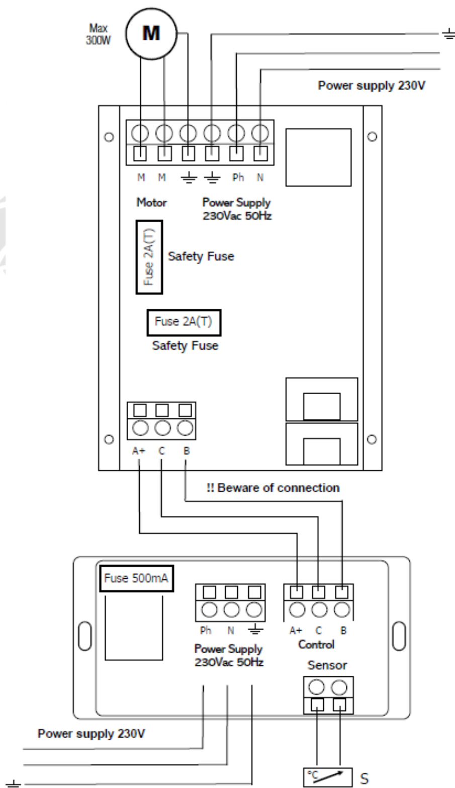
Figura nº17 - Conexiones a realizar en controlador y el módulo de potencia de la Itaca eco C/V
