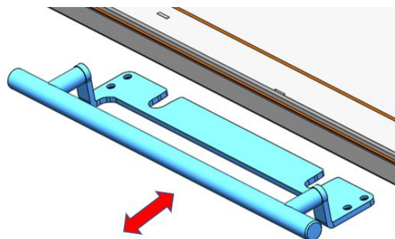
Figura n°45 - Extracción de tornillos y uso como mano fría de manilla.
