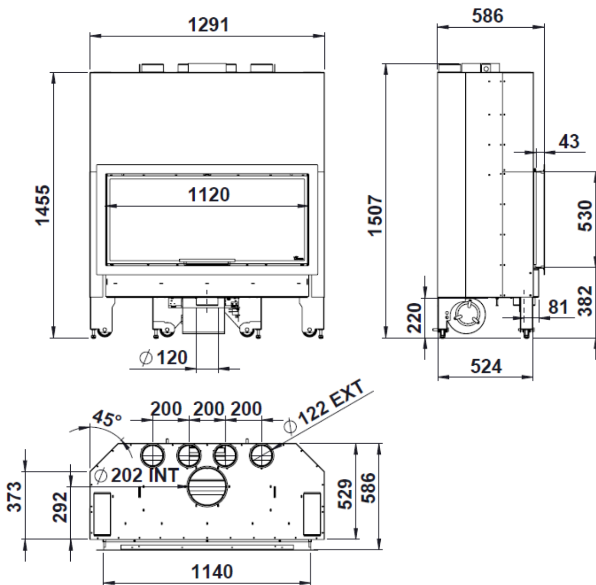
Figura n°3 - Dimensiones en mm Itaca 120 eco
