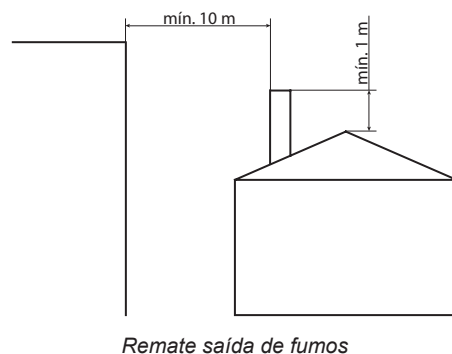
Remate saída de fumos
