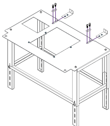
Figura 5 – Montaje de la mesa auxiliar
