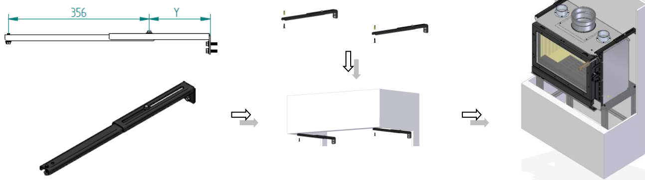
Figura 9 – Montaje de los soportes superiores - PA1090G053
