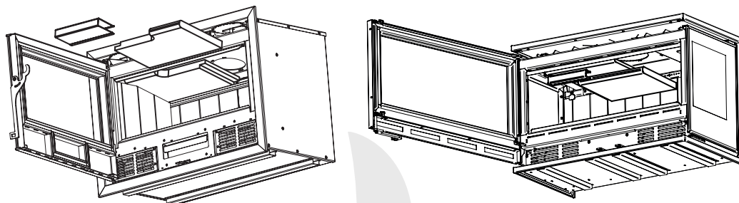
Desmontagem do defletor nos aparelhos PANORAMIC -esq.- e nos GALAXY/TAURUS -dir.-
