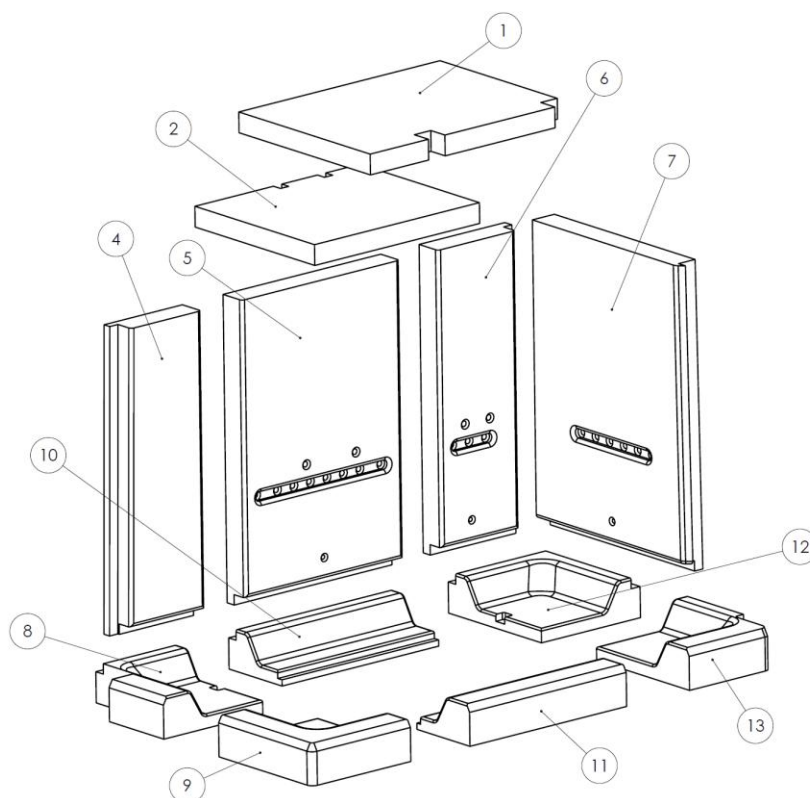
Figura nº49 - Despiece hogar vermi IZARO 80 CLI
