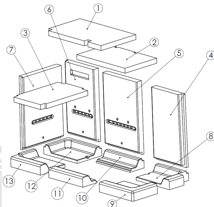
Figura nº53 - Despiece hogar vermiculita IZARO 100 CLD
