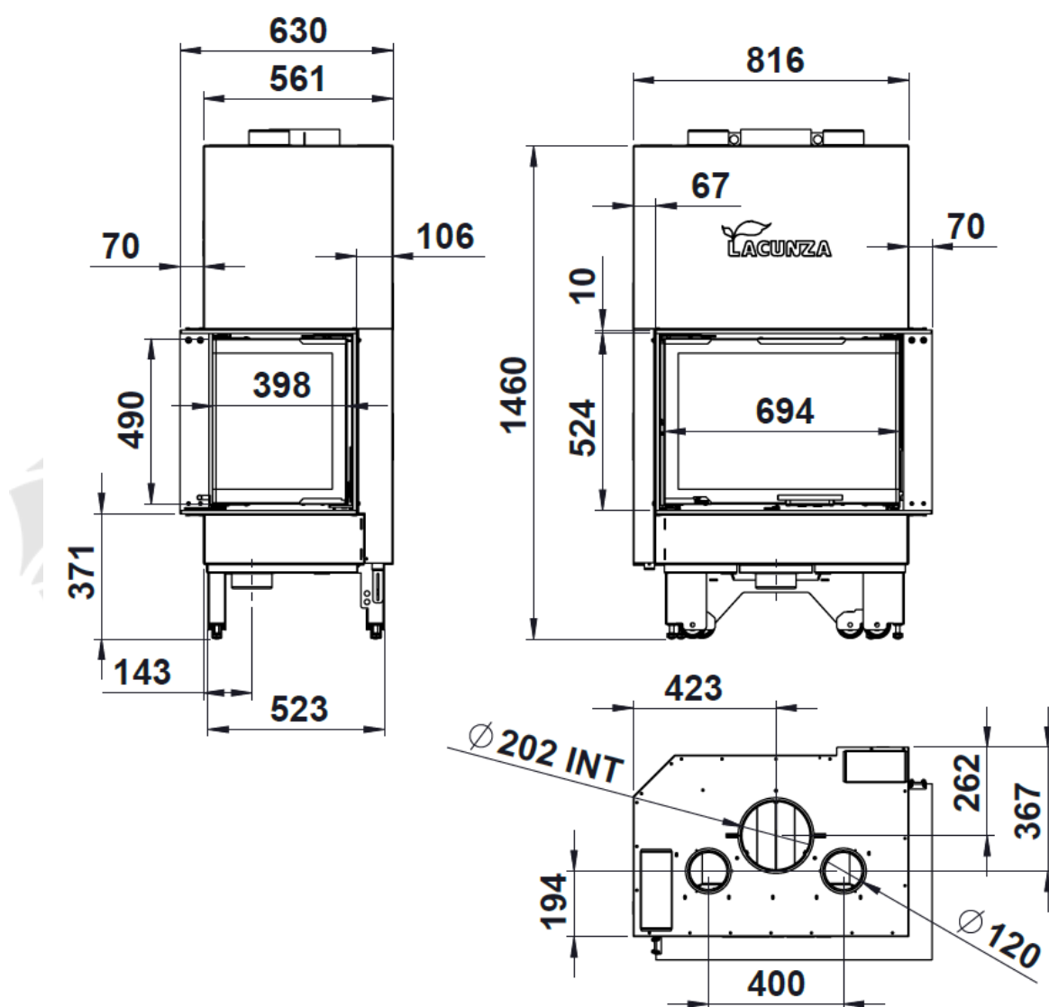
Figura nº3 - Dimensiones en mm del aparato IZARO 80 CLD
