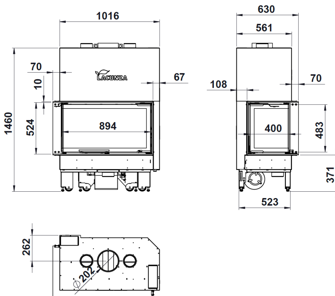
Figura nº2 - Dimensiones en mm del aparato IZARO 100 CLI
