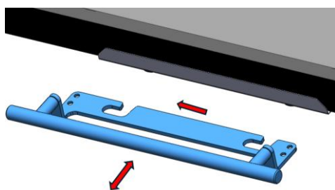
Figura nº44 - Extracción de tornillos y uso como mano fría de manilla.
