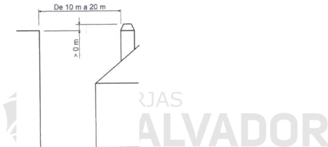
Figura nº27 - Distancias desde el remate hasta objetos entre 10 y 20m
