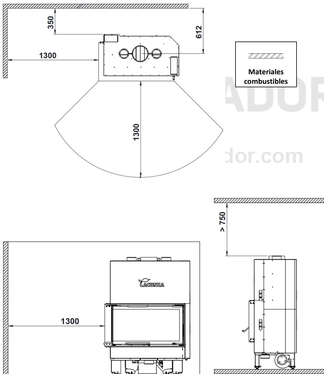
Figura nº5 - Distancias de seguridad Izaro 80-100 CLI
