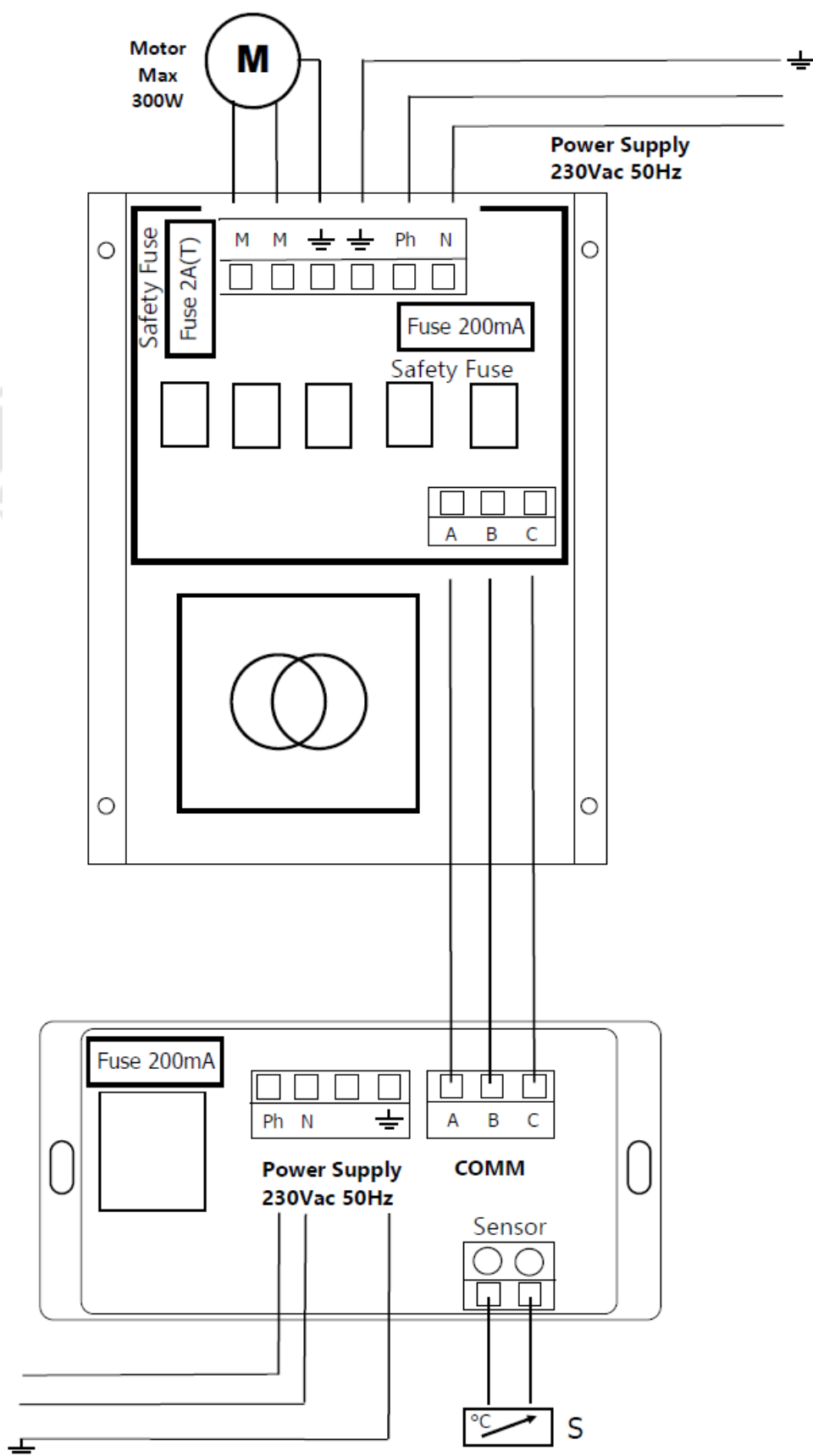
Figura n°20 - Conexiones a realizar en controlador y el módulo de potencia de la Izaro C/V
