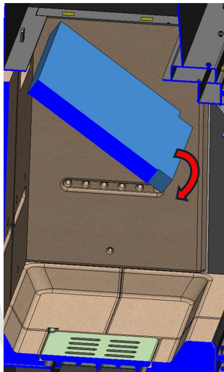
Figura nº37 - Desmontaje del deflector superior Izaro 100 CLI
