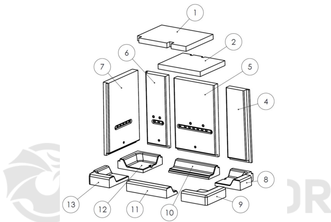
Figura nº52 - Despiece hogar vermi IZARO 80 CLD
