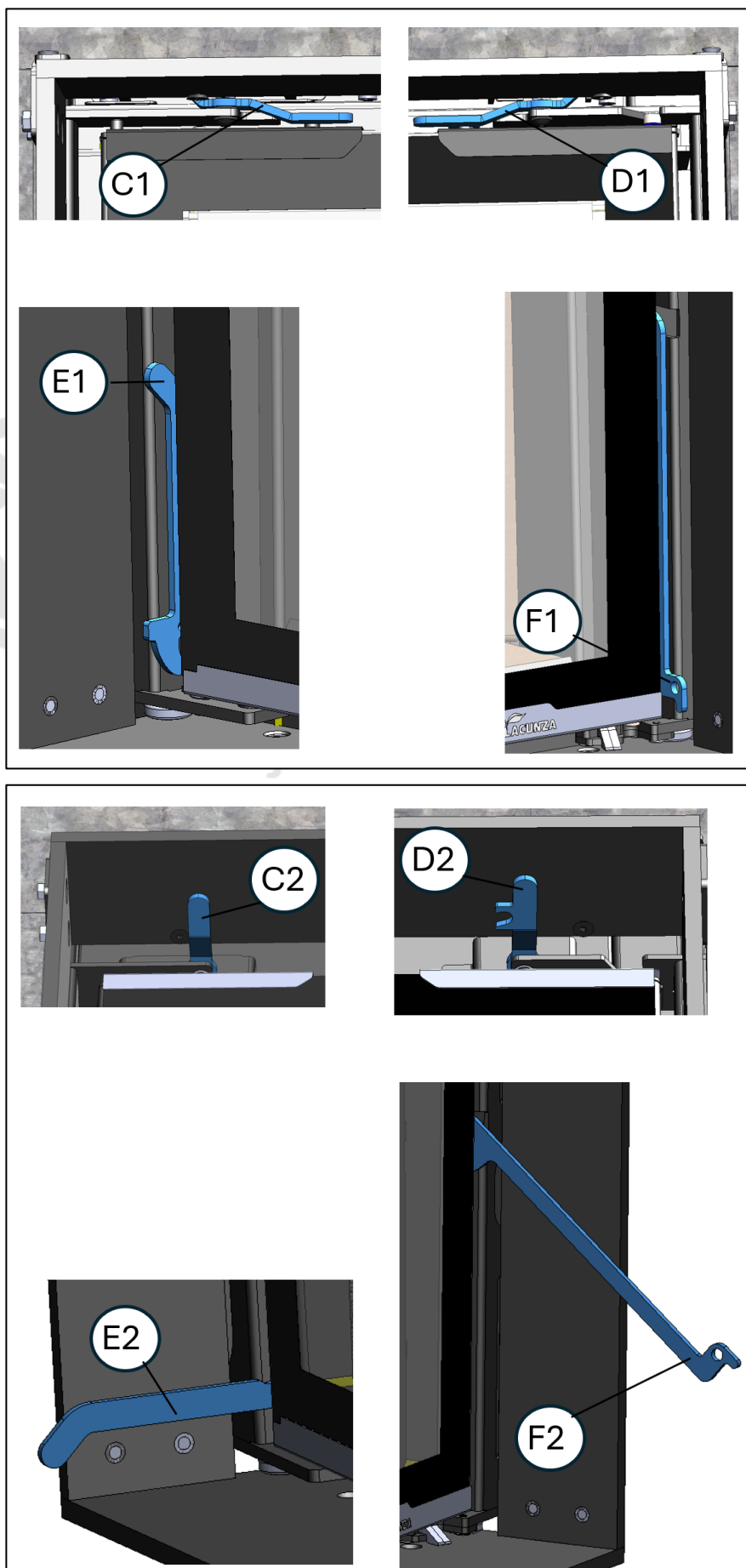
Figura nº29 - Elementos de funcionamiento del aparato IZARO 80-100 CLI
