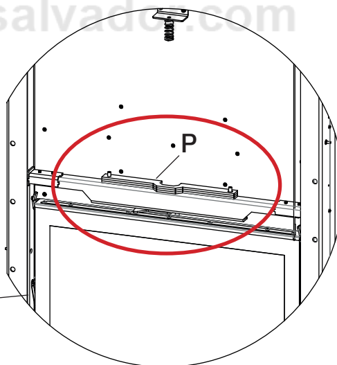
VISTA INTERNA DE LAS PLACAS SOBRE EL MARCO DE LA PUERTA
