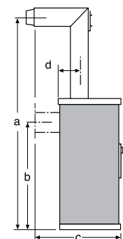
Maß a und c: mit Original-Winkelrohr dimension a and c: with original angle pipe misura a e c: con tubo ad angolo originale côtes a et c: avec conduit coudé d'origine
