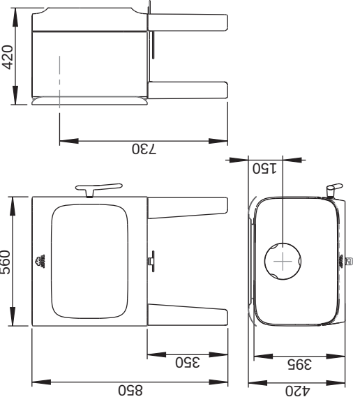
Jøtul F 305 con montanti lunghi
